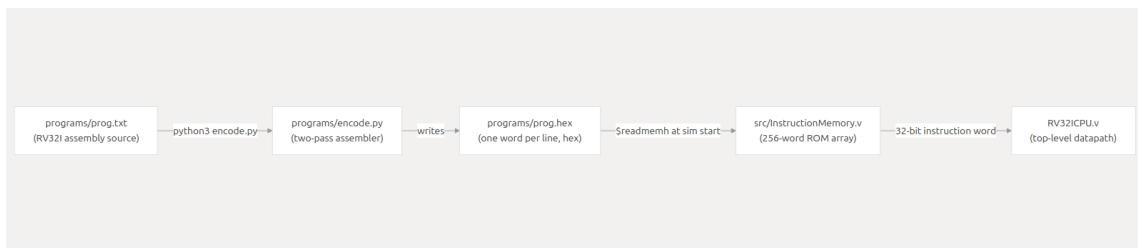
Рис. 3: Последовательность сборки hex-программы с помощью скрипта encode.py
